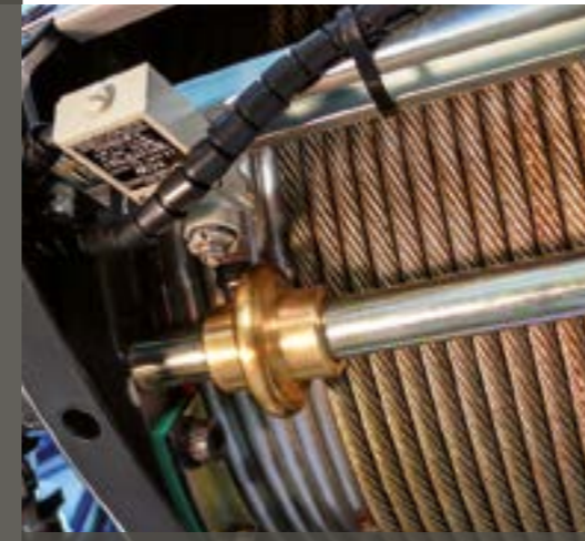
Rope guide
